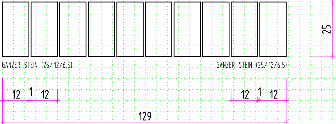
GRUNDRISS - 1. Schar
