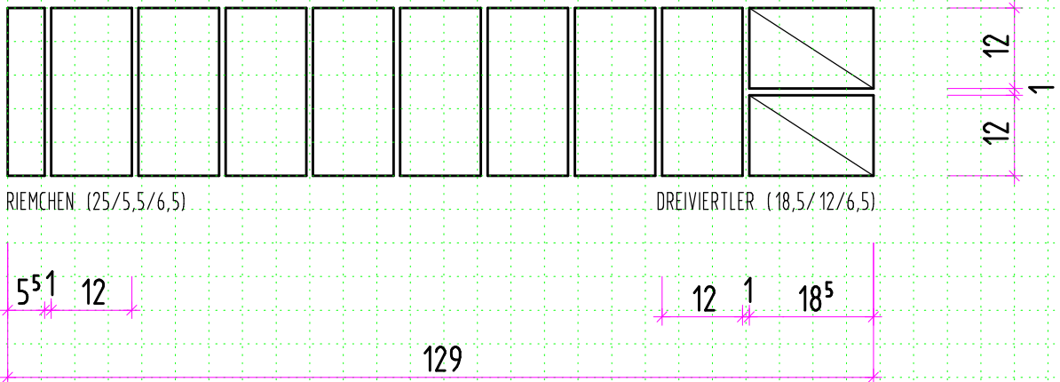
GRUNDRISS - 2. Schar
