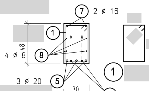
SCHNITT C-C
